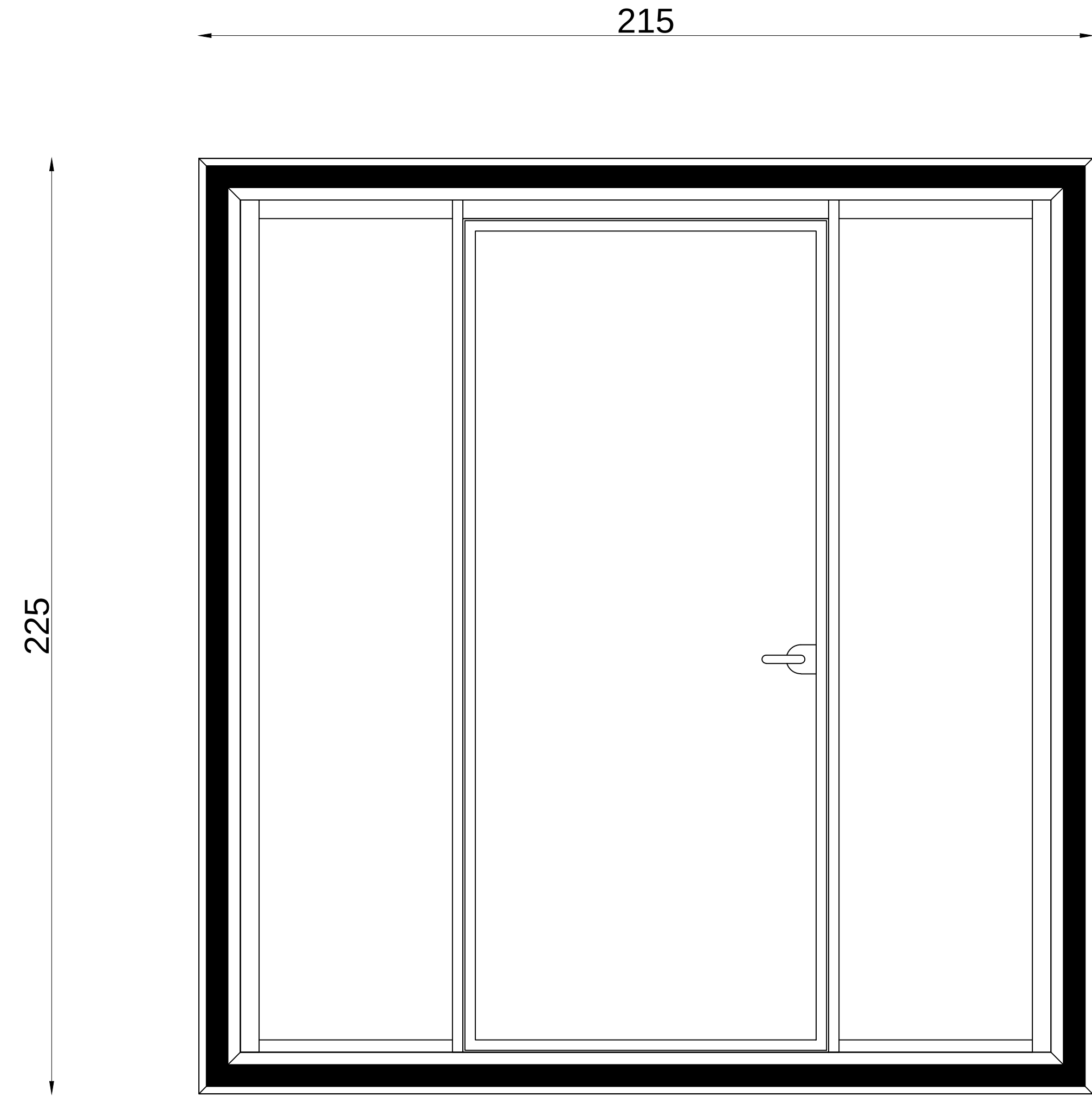
ÖN GÖRÜNÜŞ
